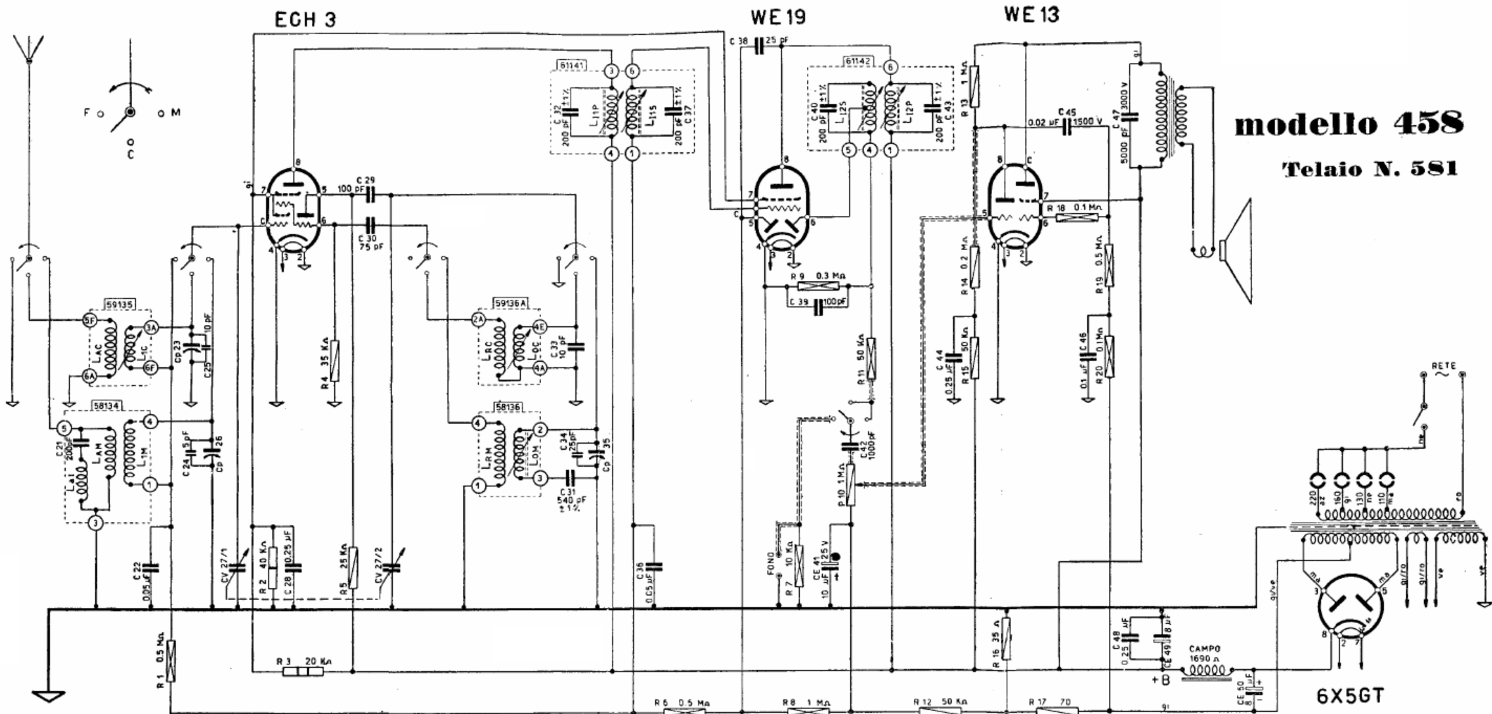
193. — LA VOCE DEL PADRONE. — Mod. 458. — Telaio 581. — Produzione 1941. — Due gamme d'onda: onde medie 192 a 580 m; onde corte 15 a 68 m. — Media frequenza: 465 kHz. — Altoparlante ellittico. — Alimentazione a corrente alternata da 100 a 200 volt, 42-60 Hertz. — Potenza d'uscita indistorta: 3 watt. — Consumo: 43 watt circa. — Peso kg. 7,5. — Dimensioni d'ingombro: cm. 37×22×21. (Tabelle tensioni e taratura v. « Radioriparazioni » II edizione).
